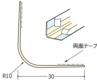
01111 S-10Rテープ付 2.5m/ミルキ- /100本入 3m/ミルキ- /100本入
