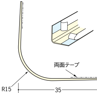
01112 S-15Rテープ付 2.5m/ミルキ- /100本入 3m/ミルキ- /50本入
