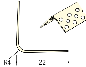
01197 S-4R穴あき 2.5m/ミルキ- /100本入 3m/ミルキ- /100本入
