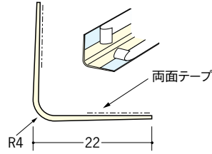
01110 S-4Rテープ付 2.5m/ミルキ- /100本入 3m/ミルキ- /100本入
