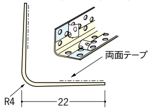
01198 S-4R穴あき+テープ付 2.5m/ミルキ- /100本入 3m/ミルキ- /100本入
