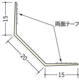
01138 面取ボードコーナー20 テープ付 2.5m/ミルキー/100本入 3m/ミルキー/100本入
