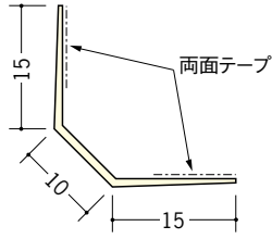
01136 面取ボードコーナー10 テープ付 2.5m/ミルキー/100本入 3m/ミルキー/100本入
