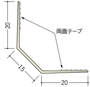
01137 面取ボードコーナー15 テープ付 2.5m/ミルキー/100本入 3m/ミルキー/100本入
