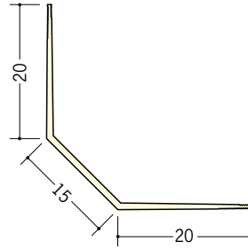
15 01042 面取ボードコーナー15 2.5m/ミルキー/100本入 3m/ミルキー/100本入
