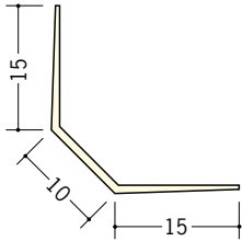
10 01041 面取ボードコーナー10 2.5m/ミルキー/100本入 3m/ミルキー/100本入
