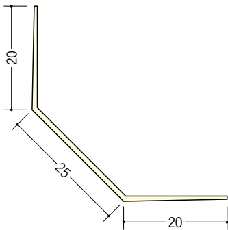
25 01036 面取ボードコーナー25 2.5m/ミルキー/50本入 3m/ミルキー/50本入
