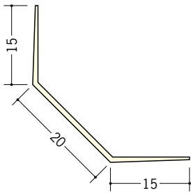
20 01043 面取ボードコーナー20 2.5m/ミルキー/100本入 3m/ミルキー/100本入
