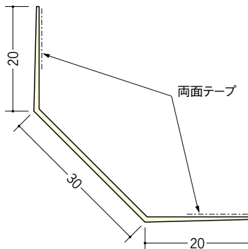
01140 面取ボードコーナー30 テープ付 2.5m/ミルキー/50本入 3m/ミルキー/50本入
