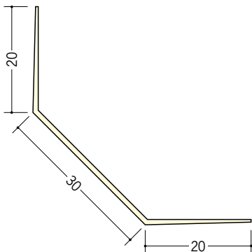
30 01044 面取ボードコーナー30 2.5m/ミルキー/50本入 3m/ミルキー/50本入
