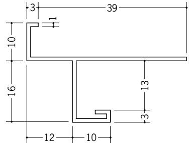
31005 見切VN-13 2m/ホワイト/80本入
