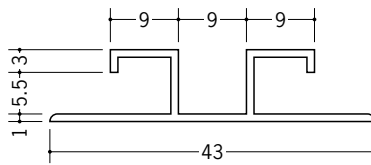
35242 ハット型EAG-5.5 2.73m/ホワイト/50本入
