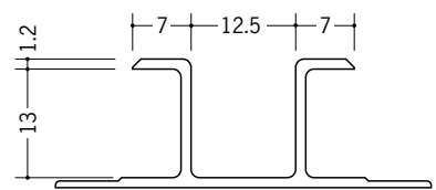
36061 ハット型12 2.5m/ホワイト 50本入
