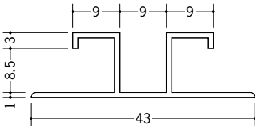
35244 ハット型EAG-8.5 2.73m/ホワイト/50本入
