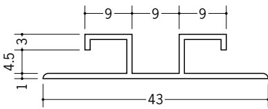
35241 ハット型EAG-4.5 2.73m/ホワイト/50本入
