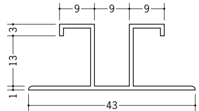
35246 ハット型EAG-13 2.73m/ホワイト/50本入
