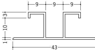
35245 ハット型EAG-10 2.73m/ホワイト/50本入
