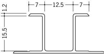
36060 ハット型15 2.5m/ホワイト 50本入
