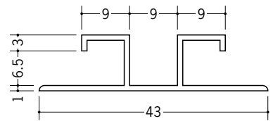
35243 ハット型EAG-6.5 2.73m/ホワイト/50本入
