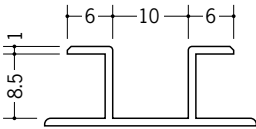
36081 ハット型8 1.82m/ホワイト 100本入
