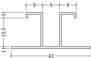
35247 ハット型EAG-15.5 2.73m/ホワイト/50本入
