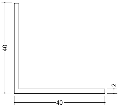
36024 アングル40 (t=2.0) 1.82m/ホワイト/40本入 2.73m/ホワイト/25本入
