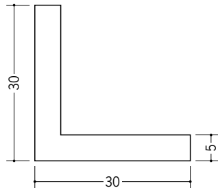
36193 アングル30 (t=5.0) 2.73m/ホワイト/15本入
