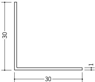
36112 アングル30 (t=1.0) 1.82m/ホワイト/100本入 2.73m/ホワイト/70本入
