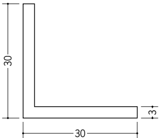
36184 アングル30 (t=3.0) 1.82m/ホワイト/30本入 2.73m/ホワイト/25本入
