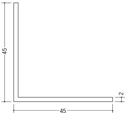
36090 アングル45 1.82m/ホワイト/20本入 2.73m/ホワイト/20本入
