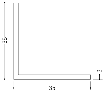
36113 アングル35 (t=2.0) 1.82m/ホワイト/50本入 2.73m/ホワイト/30本入
