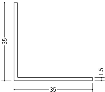
36106 アングル35 (t=1.5) 1.82m/ホワイト/50本入 2.73m/ホワイト/30本入
