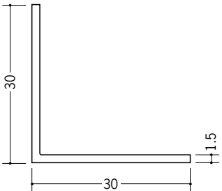
36012 アングル30 (t=1.5) 1.82m/ホワイト/100本入 2.73m/ホワイト/50本入
