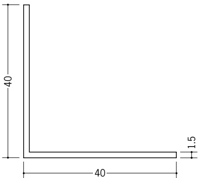
36124 アングル40 (t=1.5) 1.82m/ホワイト/50本入 2.73m/ホワイト/30本入
