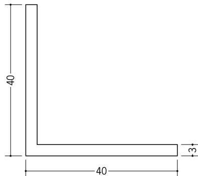
36186 アングル40 (t=3.0) 1.82m/ホワイト/25本入 2.73m/ホワイト/15本入
