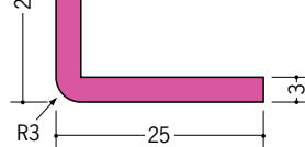
36502 カラーソフトアングル3R25×25 2.5m/軟質ビニール/各40本入 右ページの全色あり
