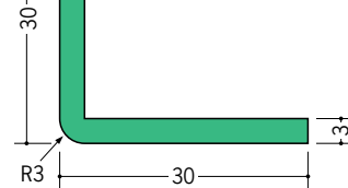
36503 カラーソフトアングル3R30×30 2.5m/軟質ビニール/各30本入 右ページの全色あり
