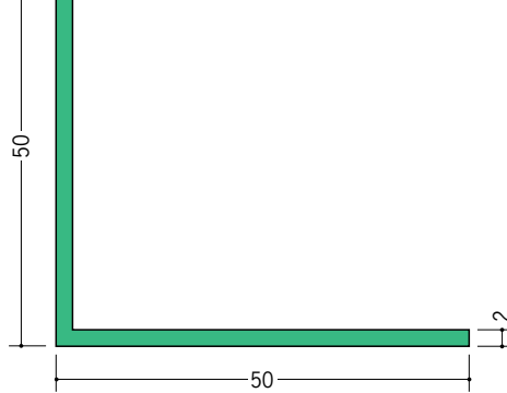
36408 カラーアングル50 2.73m/各30本入 右ページの全色あり
