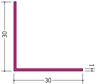
36405 カラーアングル30 2.73m/各70本入 右ページの全色あり
