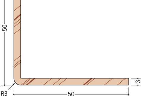
36504 カラーソフトアングル3R50×50 2.5m/軟質ビニール/各20本入 右ページの全色あり
