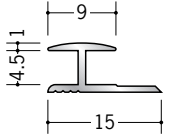
54092 アルミ4HA 1.82m/アルマイトシルバー 2.42m/アルマイトシルバー 2.73m/アルマイトシルバー
