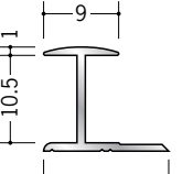
54098 アルミ10HA 1.82m/アルマイトシルバー 2.73m/アルマイトシルバー
