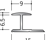
54094 アルミ6HA 1.82m/アルマイトシルバー 2.42m/アルマイトシルバー 2.73m/アルマイトシルバー
