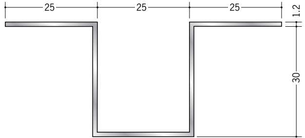
53082 アルミハット型30 3m/アルマイトシルバー
