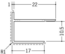
50126 アルミ10ADカラー 2.73m / バニラホワイト カスタムブラック
