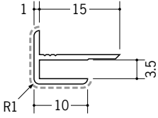
50120 アルミ3ADカラー 2.73m / バニラホワイト カスタムブラック
