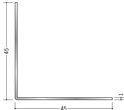
56201 アルミ折曲げ L1×45×45 3m/アルマイトシルバー
