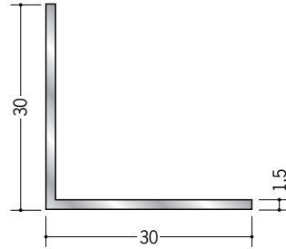
56016 アルミアングル 1.5×30×30 3m/アルマイトシルバー
