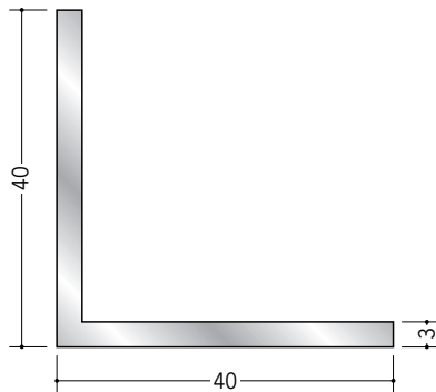
56052 アルミアングル 3×40×40 4m/アルマイトシルバー
