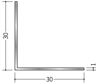
56108 アルミアングル 1×30×30 3m/アルマイトシルバー
