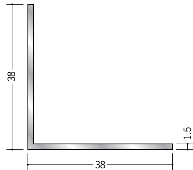
56014 アルミアングル 1.5×38×38 3m/アルマイトシルバー
