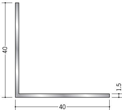
56017 アルミアングル 1.5×40×40 3m/アルマイトシルバー
