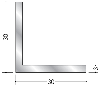
56051 アルミアングル 3×30×30 4m/アルマイトシルバー
