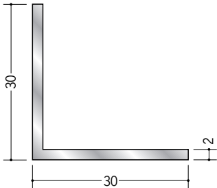
56046 アルミアングル 2×30×30 3m/アルマイトシルバー
