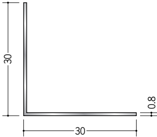
56043 アルミアングル 0.8×30×30 3m/アルマイトシルバー
