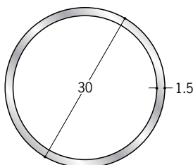
57998 アルミ丸パイプ 30×1.5 1.82m/アルマイトシルバー
