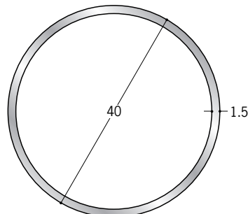
57999 アルミ丸パイプ 40×1.5 1.82m/アルマイトシルバー
