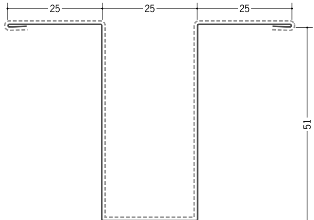
63013 カラー鉄板ハット型51 1.82m/ホワイト・クリーム/t=0.27mm
