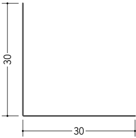
63185 L-30 1.82m/アエンメッキ鋼板 t=0.27
