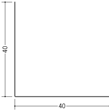
63186 L-40 1.82m/アエンメッキ鋼板 t=0.27
