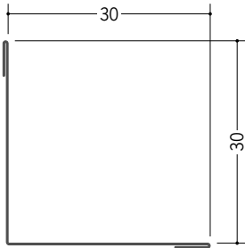
63188 L-30 (外ハゼ) 1.82m/アエンメッキ鋼板 t=0.27
