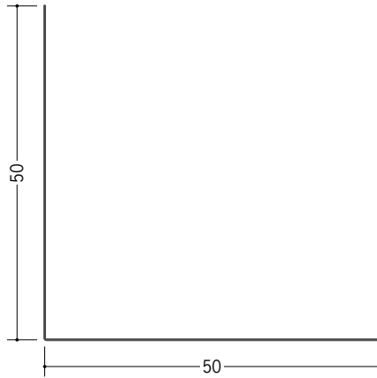
63187 L-50 1.82m/アエンメッキ鋼板 t=0.27
