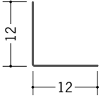
63181 L-12 1.82m/アエンメッキ鋼板 t=0.27
