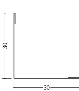
63189 L-30 (内ハゼ) 1.82m/アエンメッキ鋼板 t=0.27
