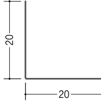
63183 L-20 1.82m/アエンメッキ鋼板 t=0.27
