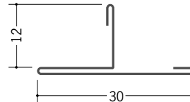
63252 TCK30-12 1.82m/アエンメッキ鋼板/t=0.27
