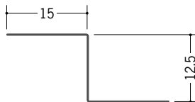
63245 水切 12 1.82m/アエンメッキ鋼板 t=0.27
