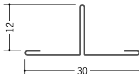
63254 TCW30-12 1.82m/アエンメッキ鋼板/t=0.27
