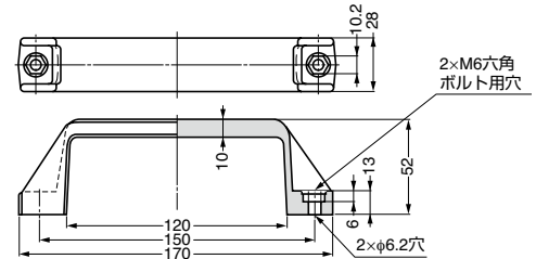
M6六角ボルト取付タイプ (大型) 213-0203
