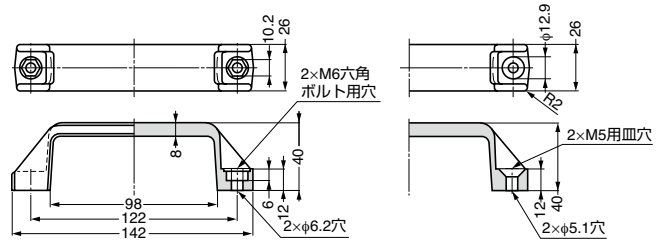
M6六角ボルト取付タイプ (小型) 213-0201
