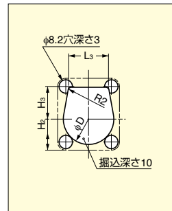
■取付加工図
