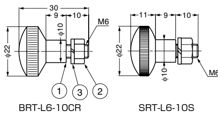
BRT-L6-10CR部品表
