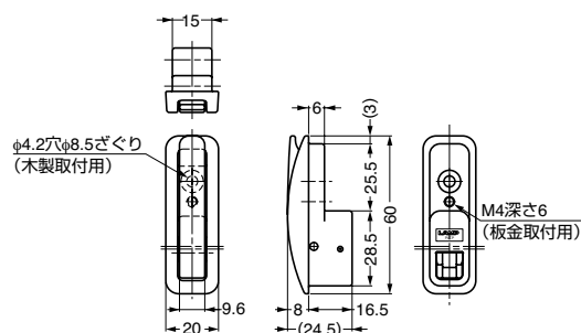
閉じた時
