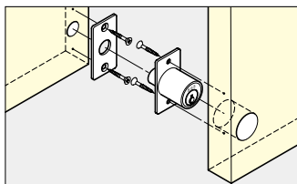
■取付仕様図
