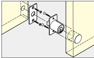
■取付仕様図
