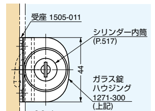
受座は、1271-200、1271-300の各中心と合わせて取り付けてください（上図は右付例）。
