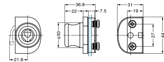
図は1271-300（右用）を示します。
