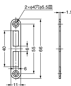
受座は、1271-200、1271-300の各中心と合わせて取り付けてください（上図は右付例）。
