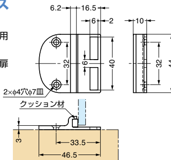
受座は、1271-200、1271-300の各中心と合わせて取り付けてください（上図は右付例）。
