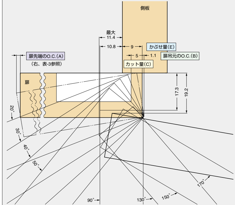
本図はカット量5mm、扉厚20mm、側板厚20mmで9mmかぶせ仕様です。
