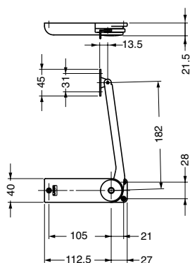
フリッパードア金具 OV-EZステア
