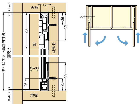
キャビネット内に扉を収納する仕様 インセット扉（扉厚19～30mmの例）
