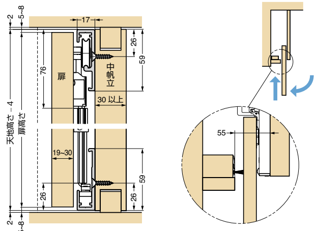
建設空間に直接取り付ける仕様 （扉厚 19～30 mm の例）
