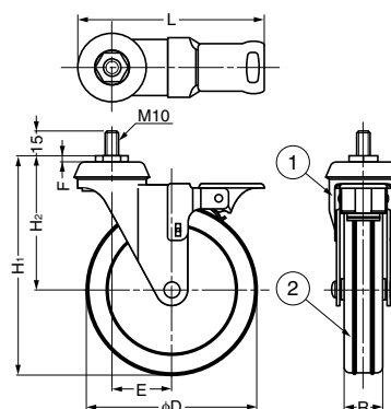
ブレーキあり (ブレーキ形状1)
