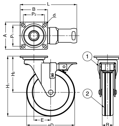
ブレーキあり (ブレーキ形状1)
