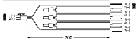
③AMPコネクタ付4本分岐ハーネス
