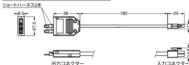
⑦HERAコネクタ付9本分岐ハーネス
