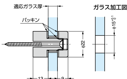
ガラス加工図
