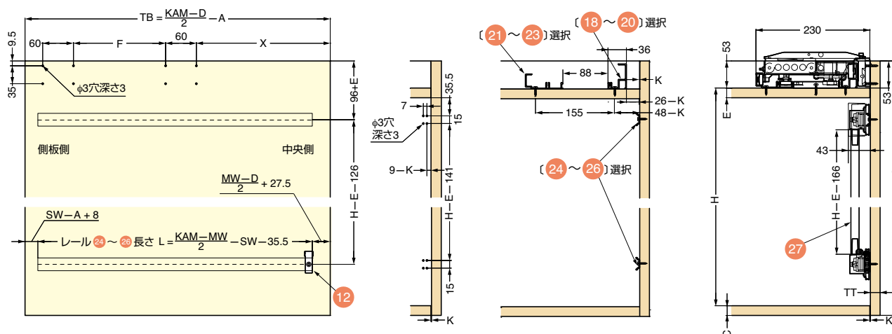
M-M' 断面図
