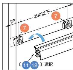
レールが側板にかぶらない場合
