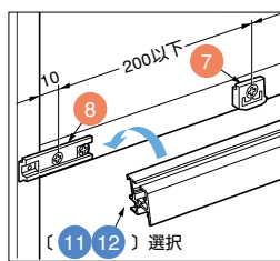
レールが側板にかぶる場合
