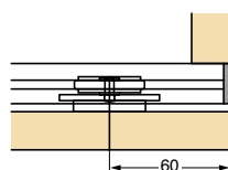
レールが側板にかぶる場合
