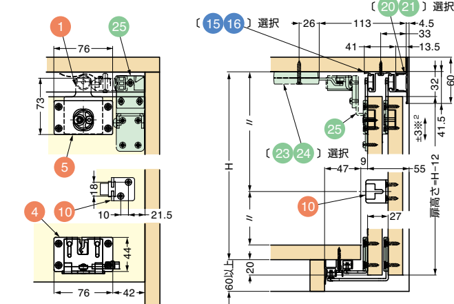
■扉の加工寸法
