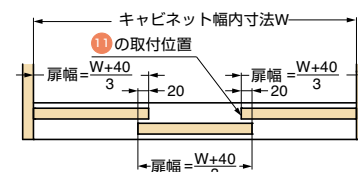
3枚扉の場合
