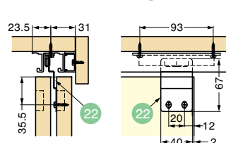
3枚扉用ストッパー ㉒取付位置
