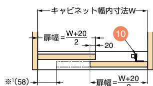
2枚扉の場合
