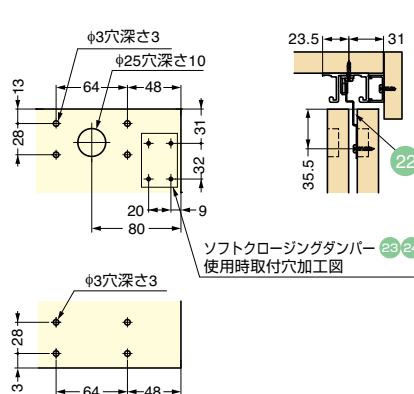
■扉の加工寸法
