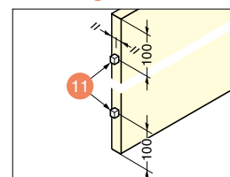
■扉の高さ調整
