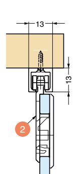
上レール (シングル面付用) ⑩⑪使用時
