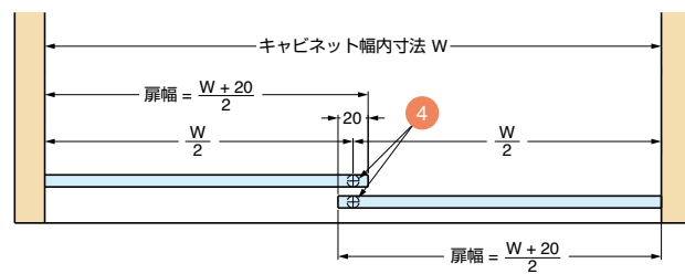
上レール (ダブル掘込用) ⑧⑨使用時
