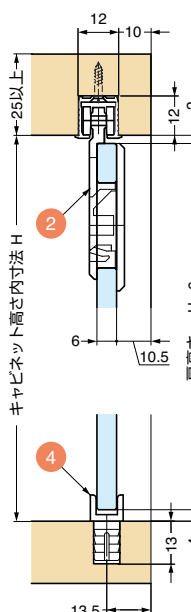
上レール (シングル掘込用) ⑥⑦使用時
