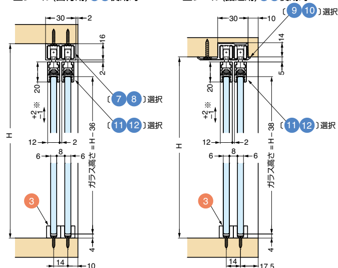
上レール (面付用) ⑦⑧使用時
