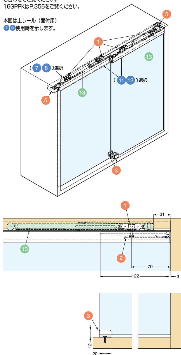
上レール (面付用) ⑦⑧使用時
