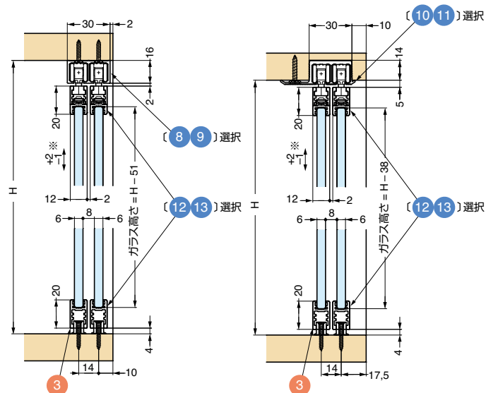
上レール (面付用) ⑧⑨使用時
