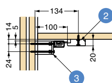
■側断面図
