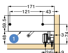
■上面図
