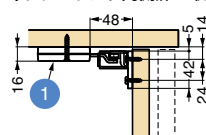
■側断面図
