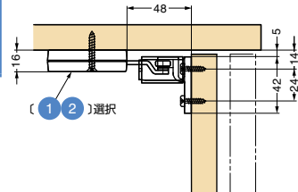
■側断面図(キャビネット内側扉に取り付ける場合)
