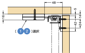
■側断面図(キャビネット外側扉に取り付ける場合)
