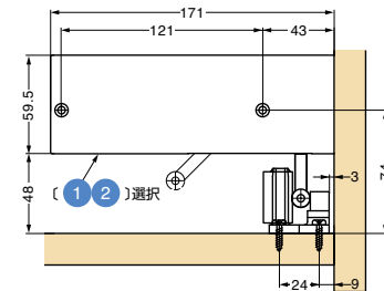
■側断面図(キャビネット内側扉に取り付ける場合)
