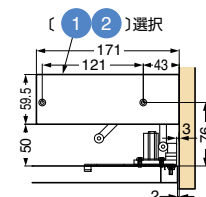
■上面図
