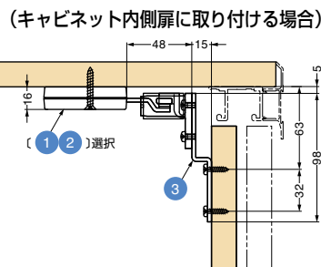
■側断面図
