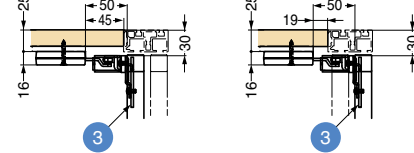
（キャビネット内側扉に取り付ける場合） （キャビネット外側扉に取り付ける場合）
