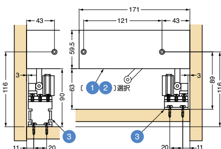
■上面図
