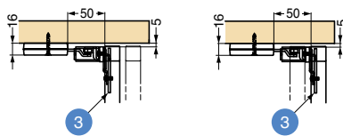
（キャビネット内側扉に取り付ける場合） （キャビネット外側扉に取り付ける場合）
