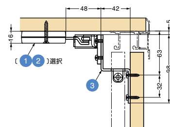
（キャビネット外側扉に取り付ける場合）
