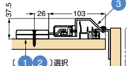
■側断面図
