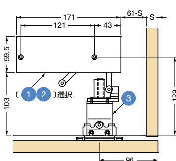
■上面図
