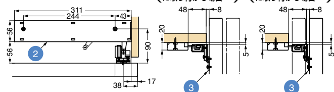
■上面図
