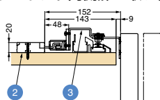
■側断面図
