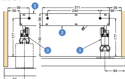
■上面図
