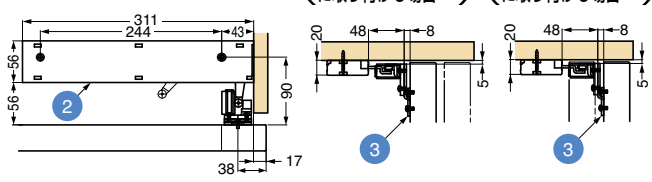
■上面図
