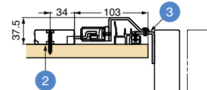
■側断面図
