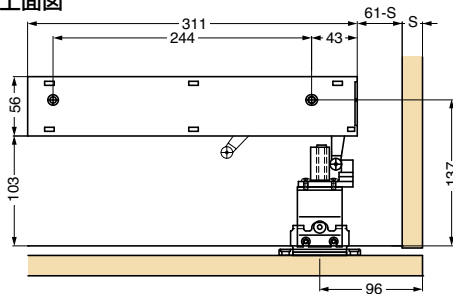
■上面図
