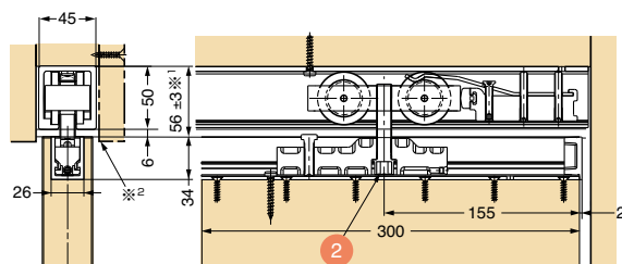
下ガイドレール (12) 使用例
