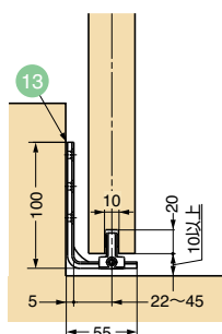
壁付ガイド (13) 使用例
