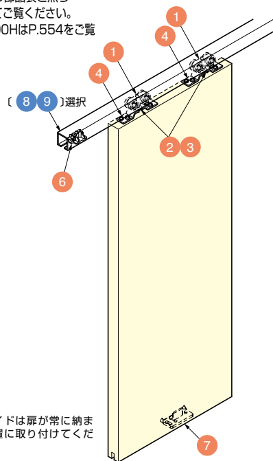
天付仕様
