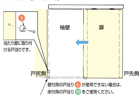
壁付仕様
