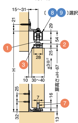
壁付仕様
