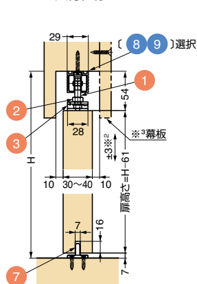
天付仕様
