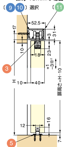
幕板(11・12)使用時 扉厚40mmの場合
