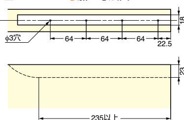
木製幕板使用時 扉厚40mmの場合
