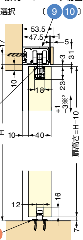
木製幕板使用時 扉厚40mmの場合
