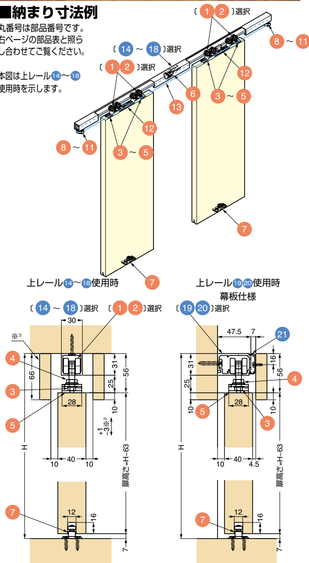
ハンガーパーツ(5)、シンクロブラケット(12)取付位置
