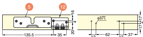
ハンガーパーツ(5)、シンクロブラケット(12)取付位置
