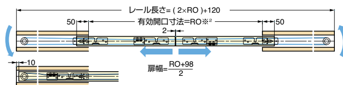
ハンガーパーツ(5)、シンクロブラケット(12)取付位置
