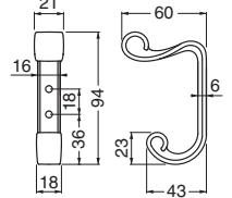
CZ-23 フレイジュ帽子掛 (亜鉛合金/A3.5×20)
