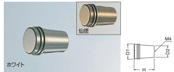
KB-97 ピルツツマミ (真チュウ/ISO4×28)
