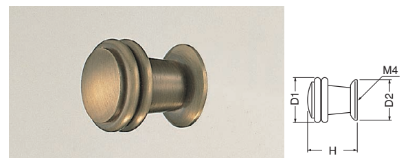
KB-86 サーフツマミ (真チュウ/ISO4×28)
