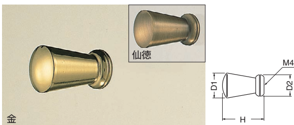
KB-94 チェストツマミ (真チュウ/ISO4×28)
