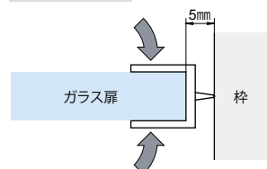
取付説明図
