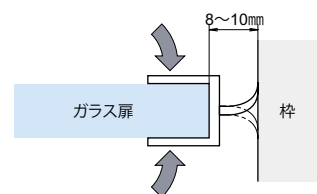
取付説明図
