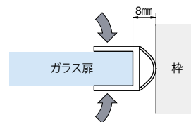
取付説明図
